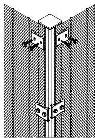
DETAIL HOEKPAAL
