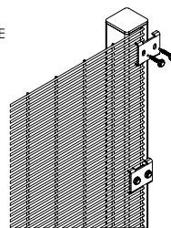
DETAIL EINDPAAL
