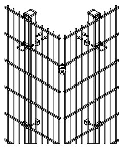
DETAIL HOEKPAAL
