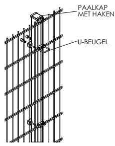
DETAIL TUSSENPAAL
