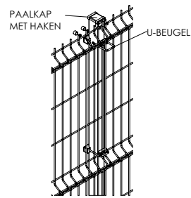
DETAIL EINDPAAL
