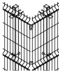
DETAIL HOEKPAAL
