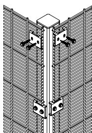
DETAIL HOEKPAAL
