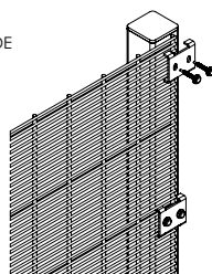
DETAIL EINDEPAAL
