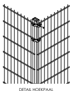
DETAIL HOEKPAAL
