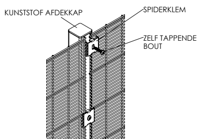
DETAIL TUSSENPAAL
