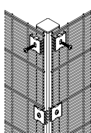
DETAIL HOEKPAAL
