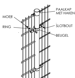
DETAIL TUSSENPAAL
