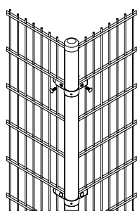
DETAIL HOEKPAAL
